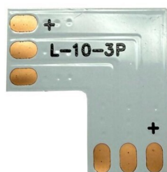
Łącznik Kątowy L CCT 10mm 3 Piny ES-LA-303
